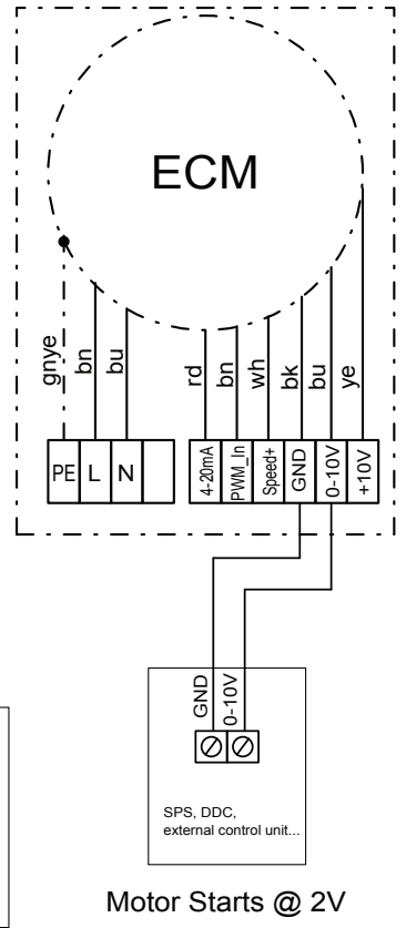
Připojení signálu 0-10V
